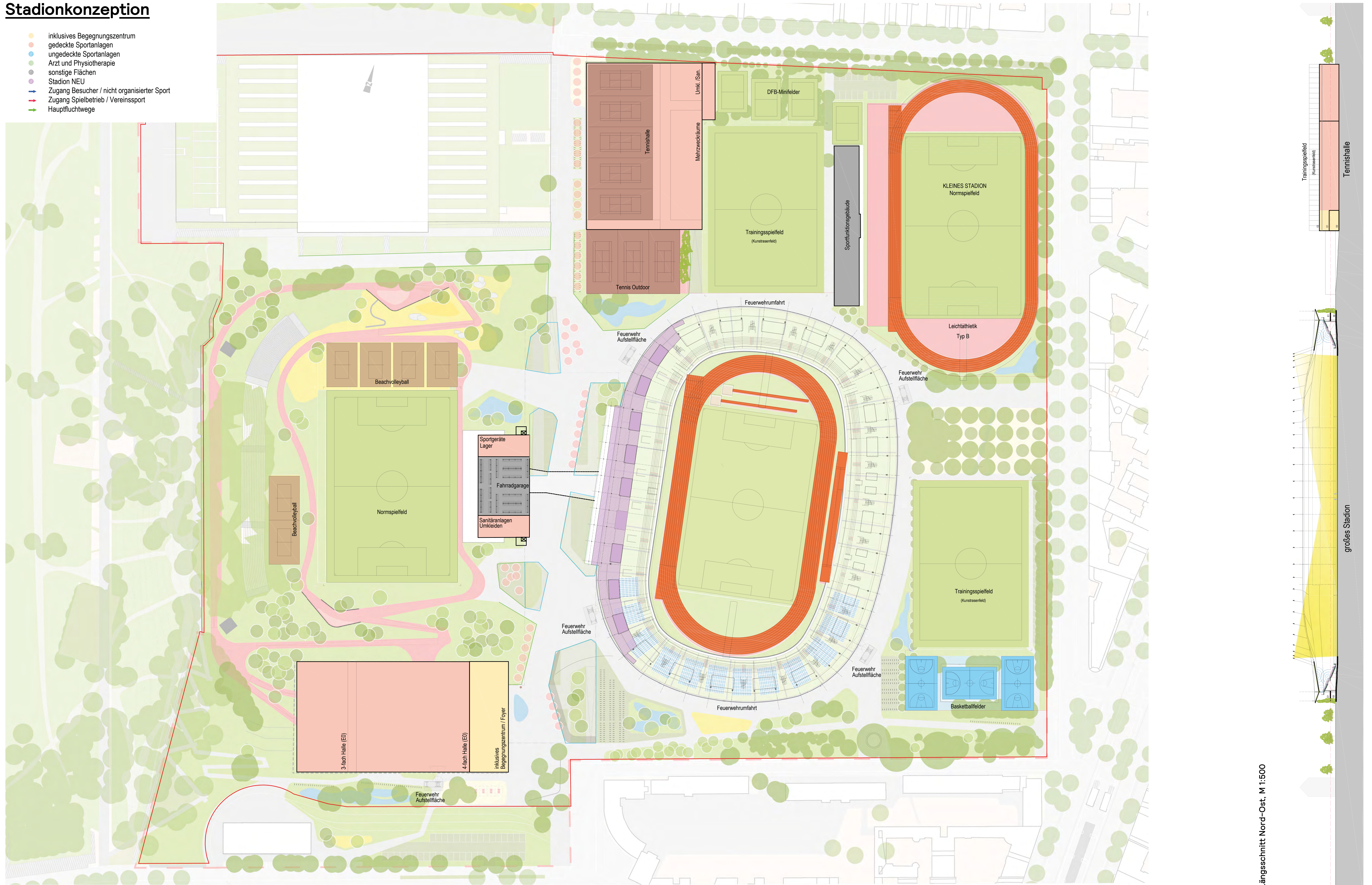
Lageplan Ebene E1, M 1:1000
