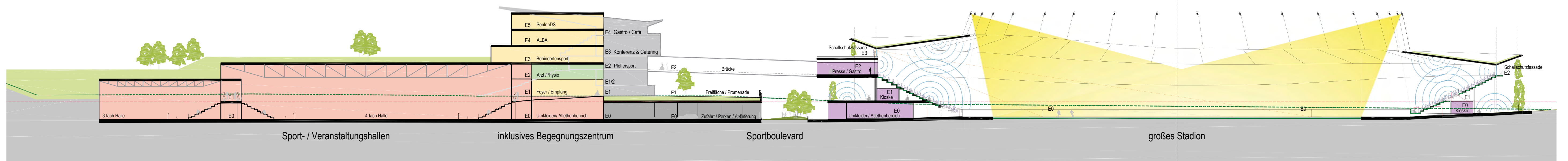
Längsschnitt Ost-West, M 1:500
